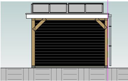
Rechtergevel
