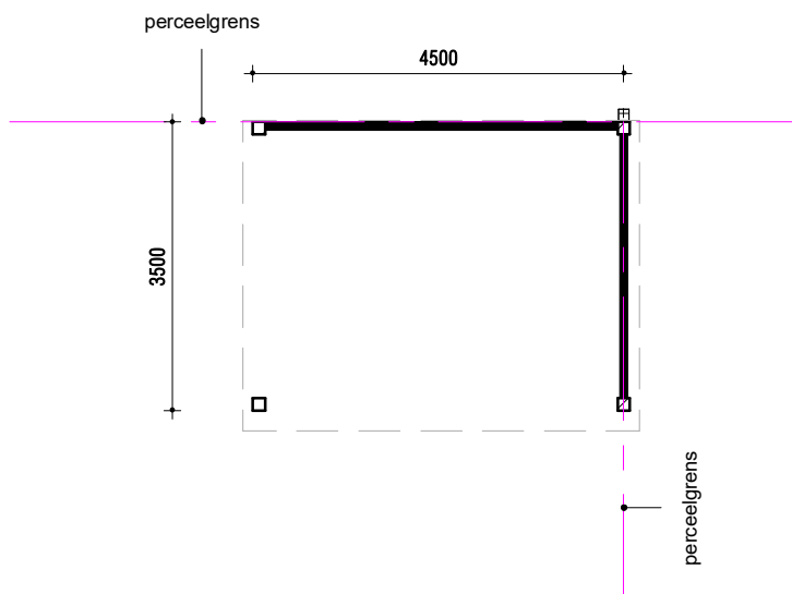
Begane grond
