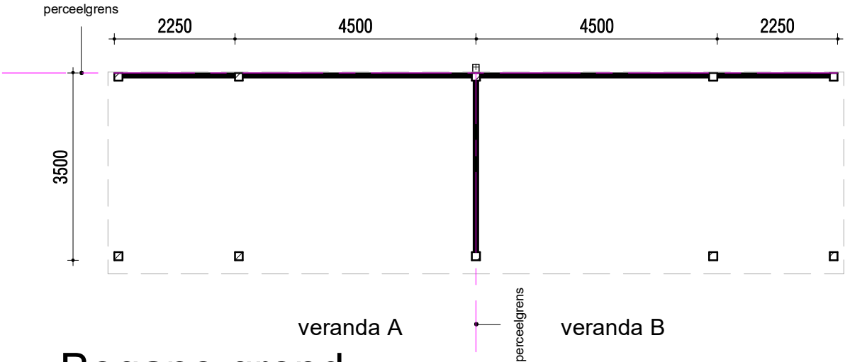
Begane grond
