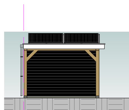
veranda A Linkergevel
