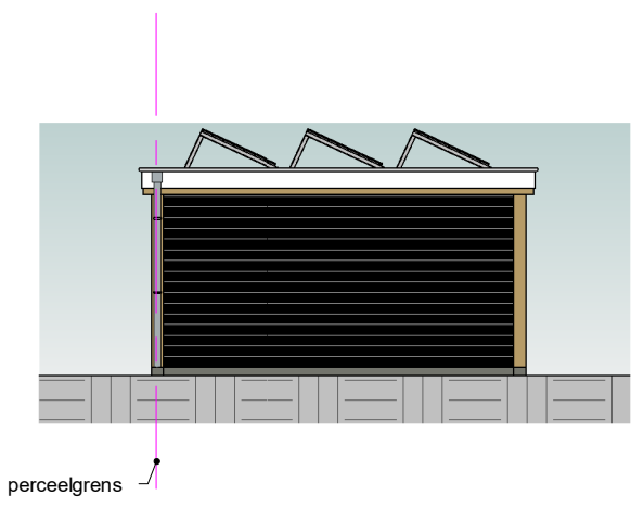
Achtergevel
