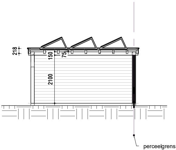
Doorsnede
