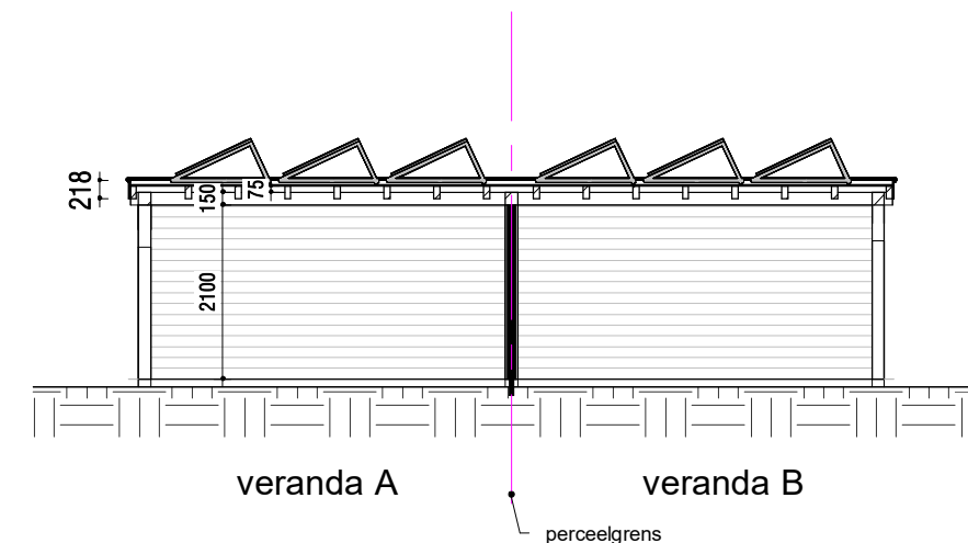
Doorsnede
