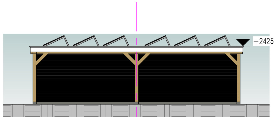
veranda A veranda B Voorgevel
