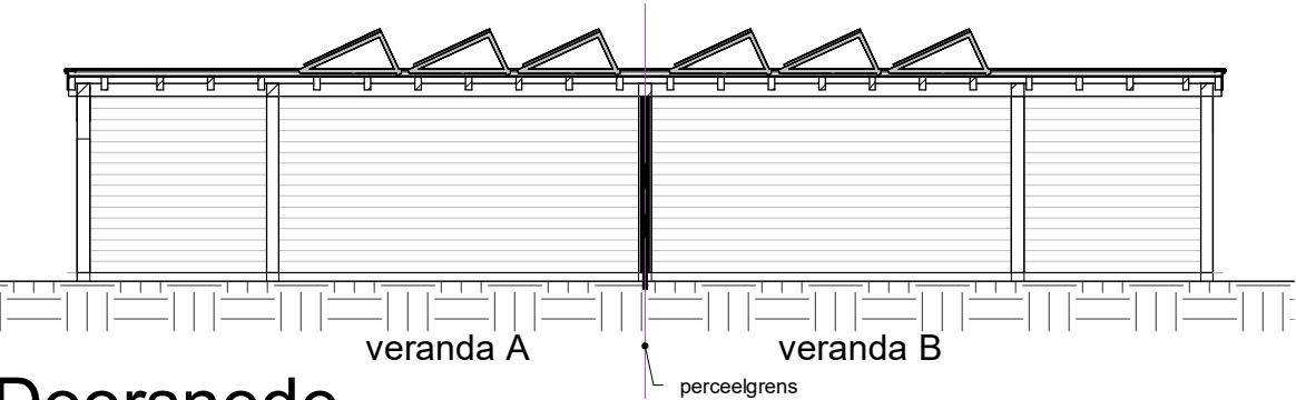
Doorsnede
